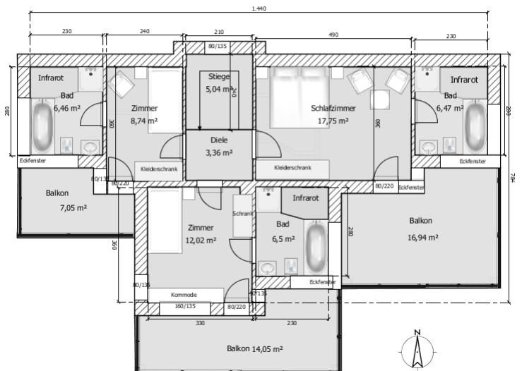
OBERGESCHOSS ca.64m 2
