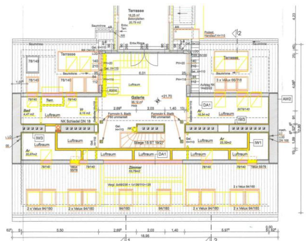
GALERIEGESCHOSS
