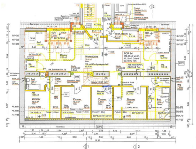
DACHGESCHOSS
